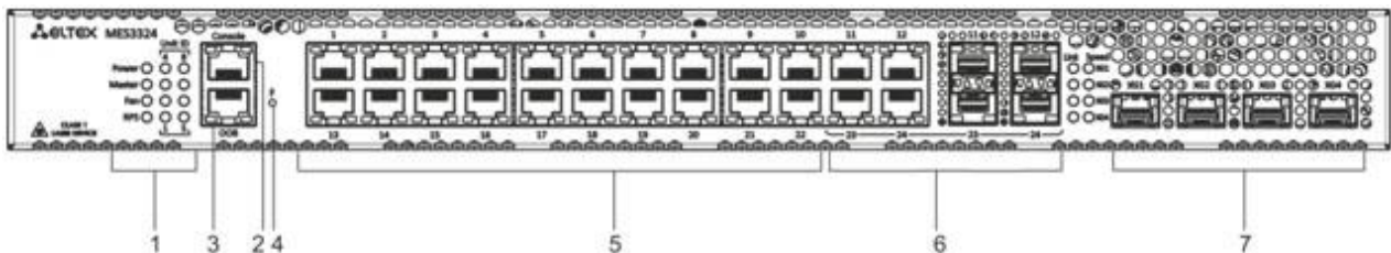
Рисунок 3 — Передняя панель MES3324
